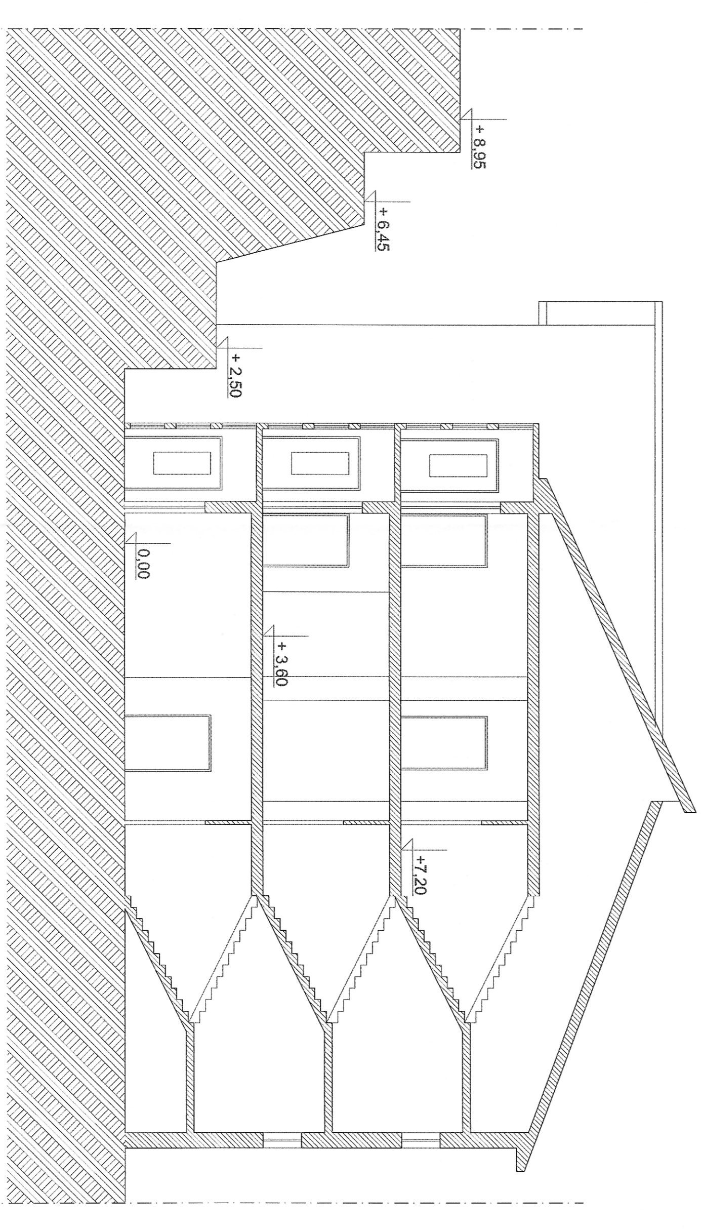
SEZIONE TRASVERSALE B-B' - Riqualificazione
