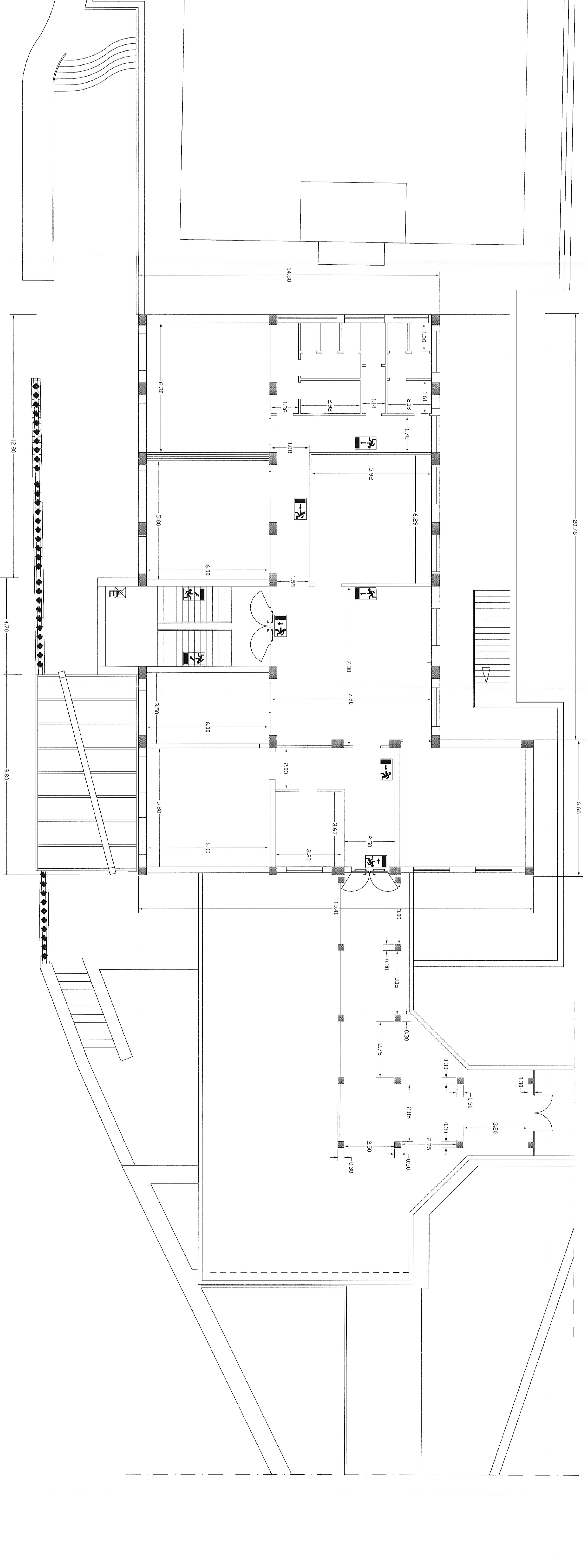
PIANTA TERZO LIVELLO - Stato di Attuale
